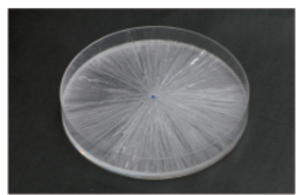
塩化アンモニウム結晶が雪のように積もる様子を観察! 核となるビーズを落とし、酢酸ナトリウムが結晶に!
