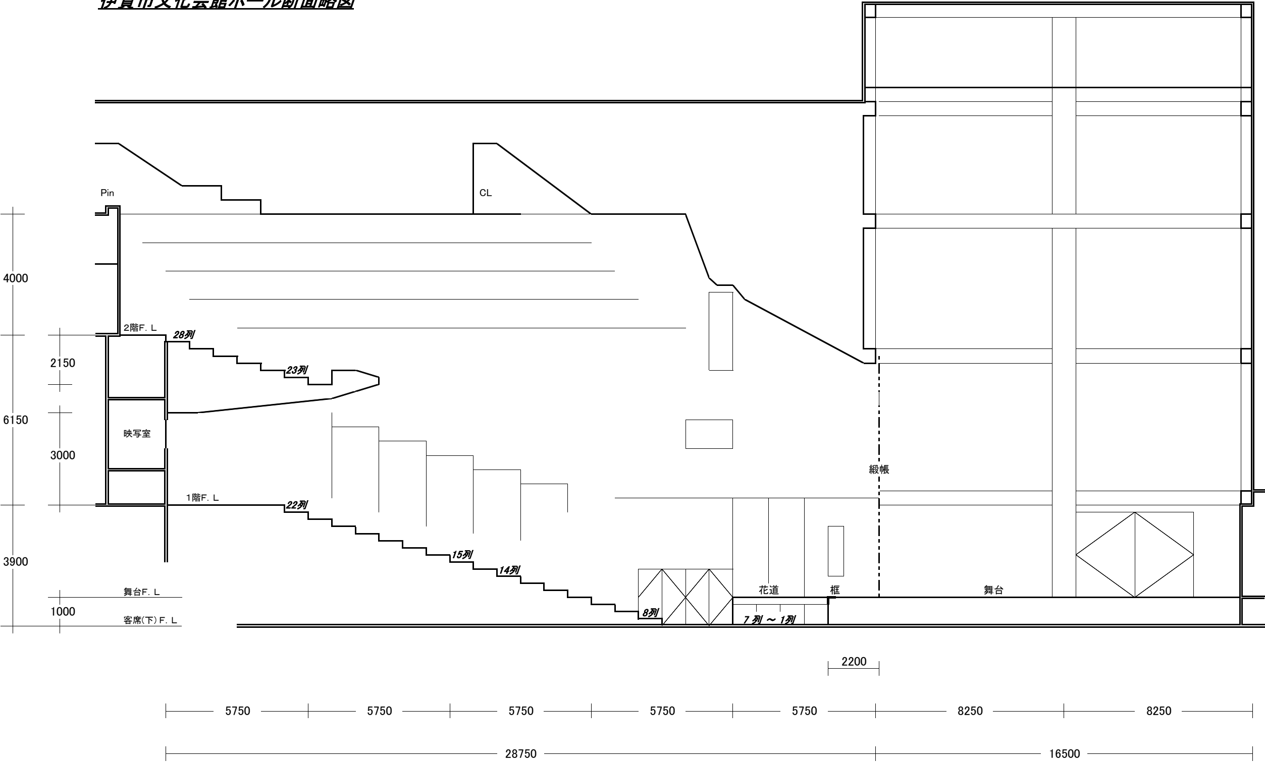
伊賀市文化会館ホール断面略図
